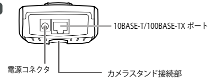
底面
