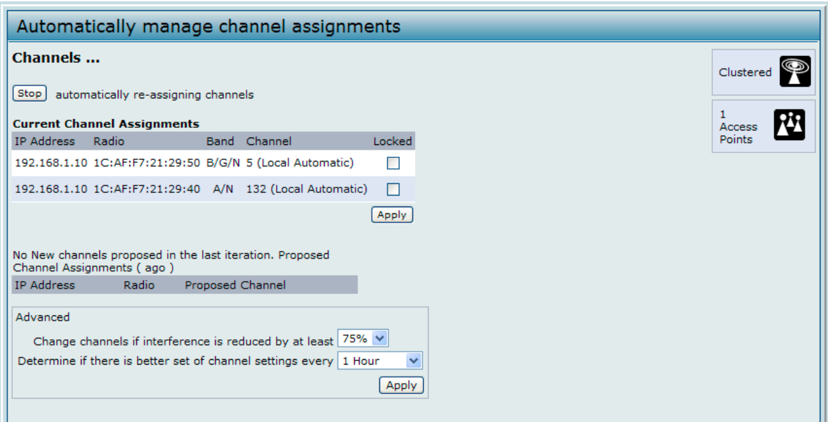
図 10-6 チャンネル割り当ての管理 画面 - 自動チャンネル割り当て有効
