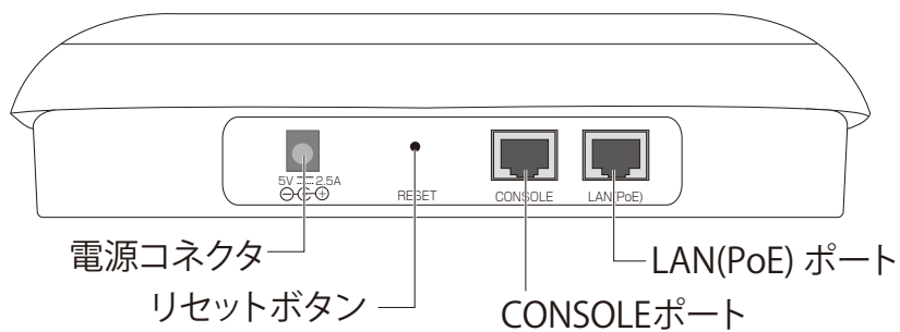
図 1-4 上面パネル図（DWL-3600AP）
