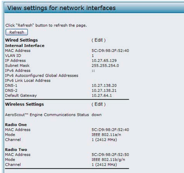
図 4-1 ネットワークインタフェースの設定参照 画面
