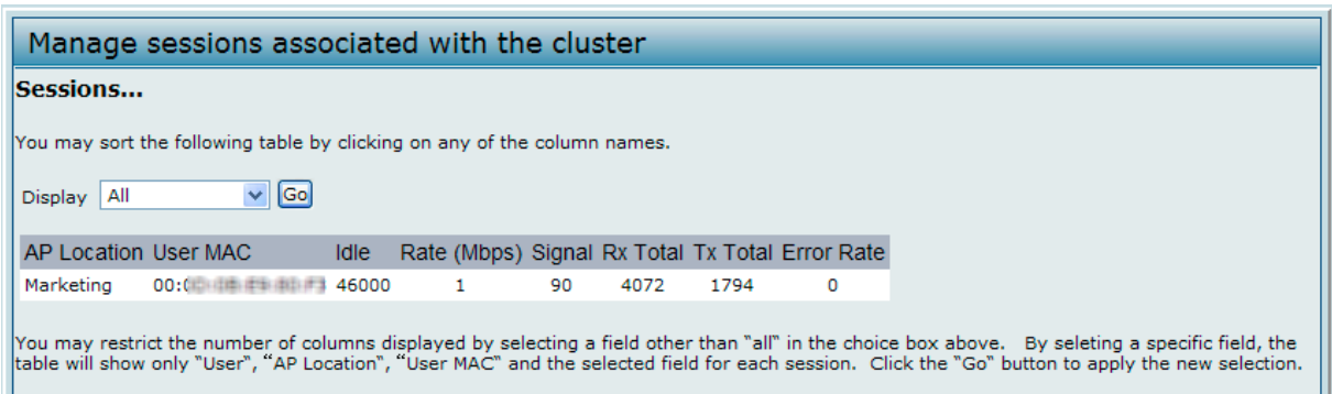
図 10-4 クラスタに接続するセッションの管理画面 - セッションあり
