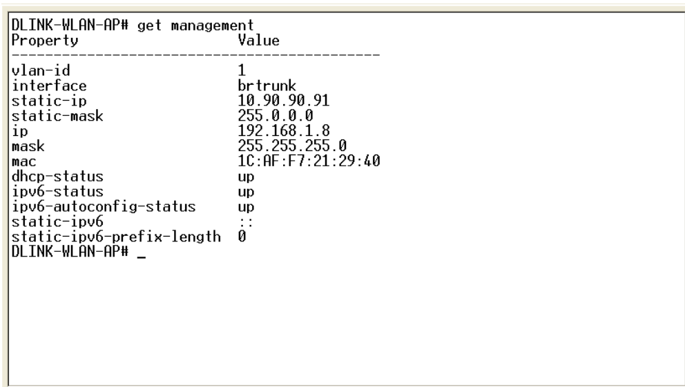
図 3-4 get management 画面
