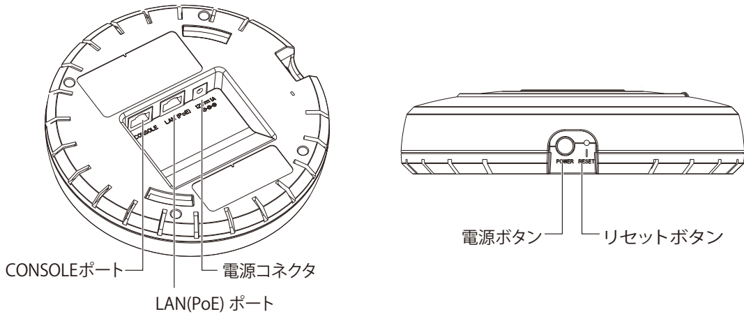
図 1-2 底面 / 側面パネル図（DWL-2600AP）
