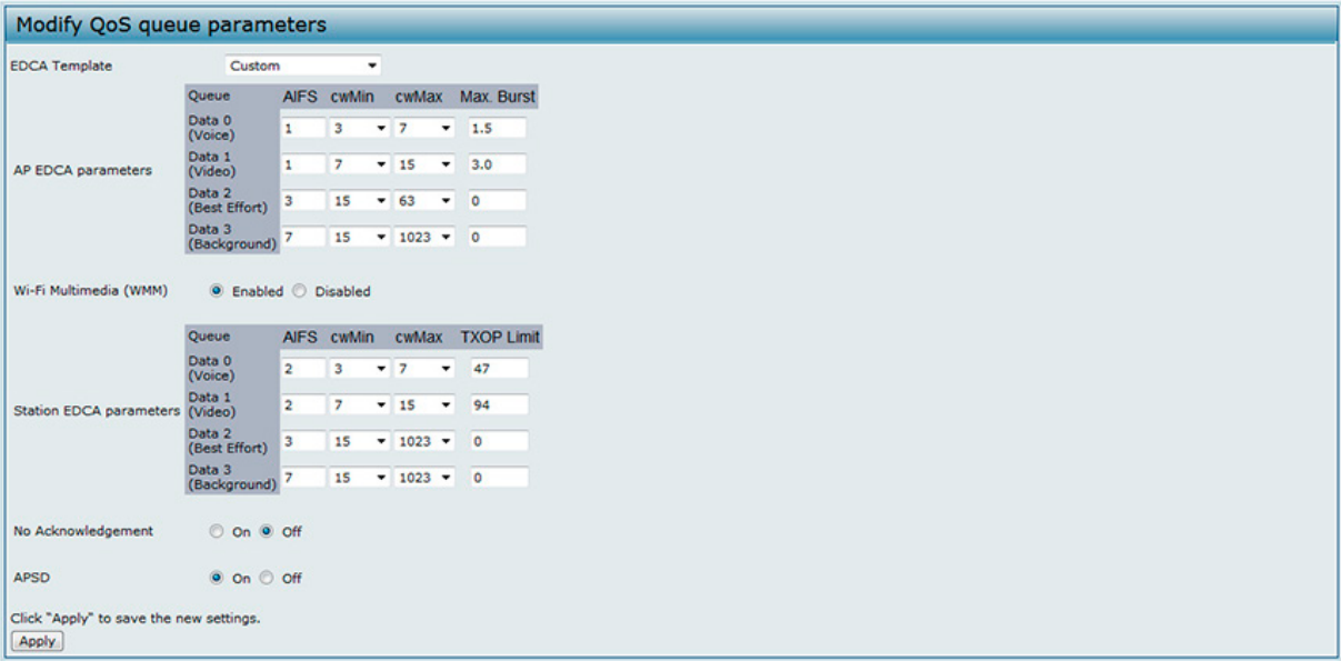
図 6-5 QoS キューパラメータの設定 画面
