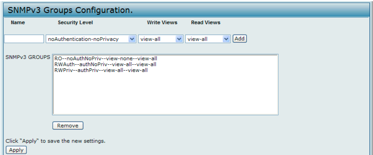
図 7-2 SNMPv3 グループの設定 画面
