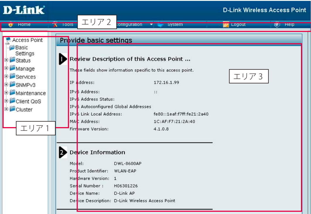
図 3-6 Web マネージャのメイン画面
