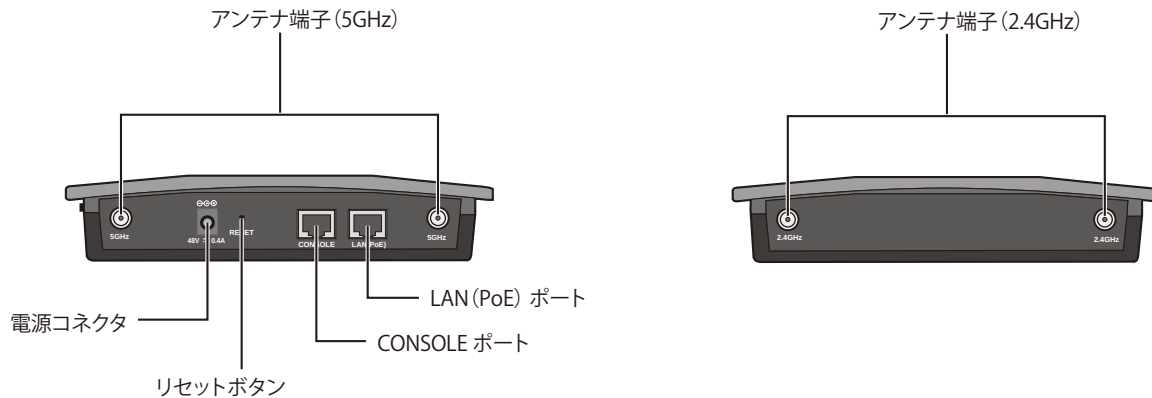
図 1-8 上面、下面パネル図（DWL-8600AP）
