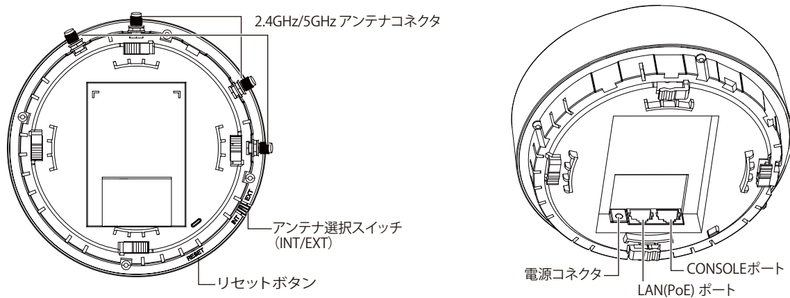
図 1-6 底面パネル図（DWL-6600AP）
