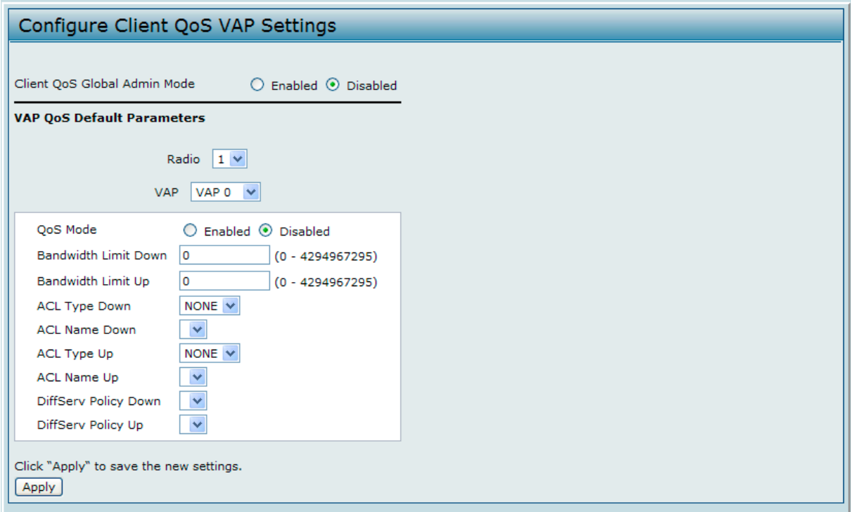
図 9-1 クライアント QoS の VAP 設定 画面
