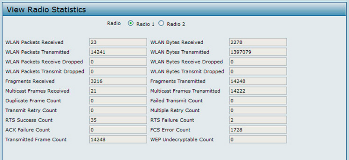
図 4-14 Radio Statistics 画面
