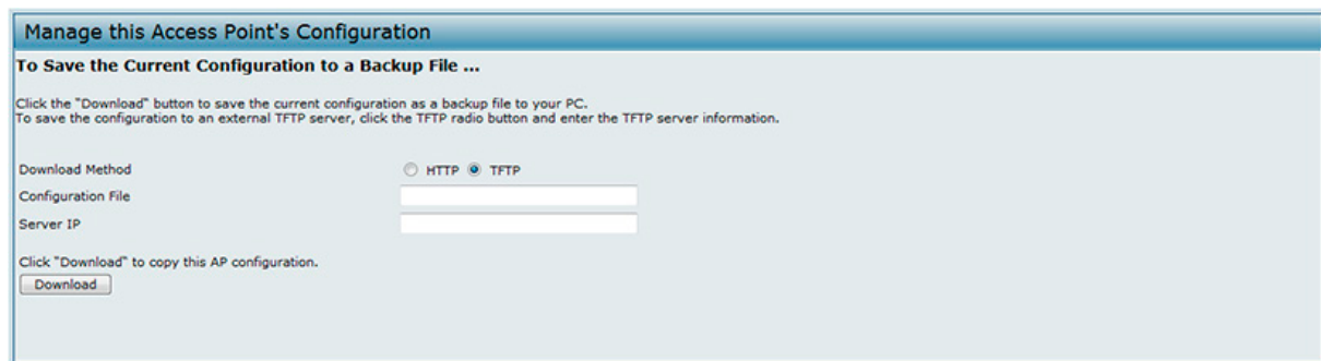
図 8-1 アクセスポイントのコンフィグレーションの管理画面 - 保存
