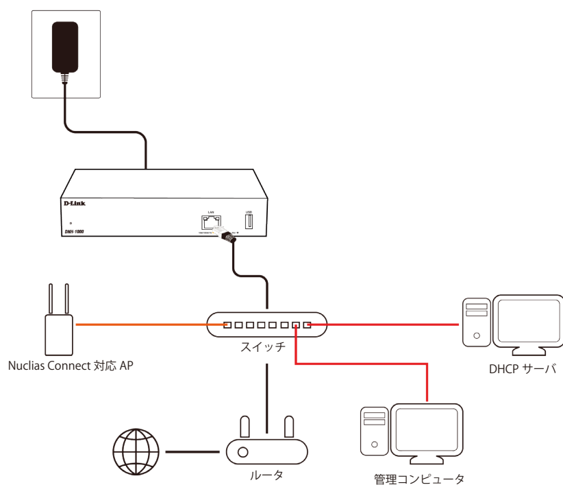
図 3-1 接続例
