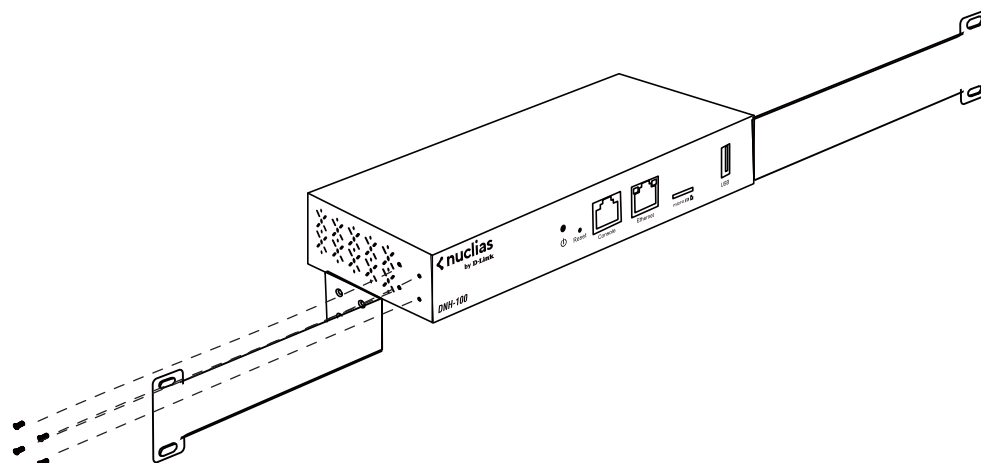
図 2-1 ゴム足の取り付け
