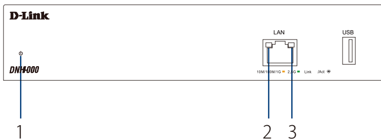
図 1-3 DNH-1000 の LED 配置図 (前面パネル)
