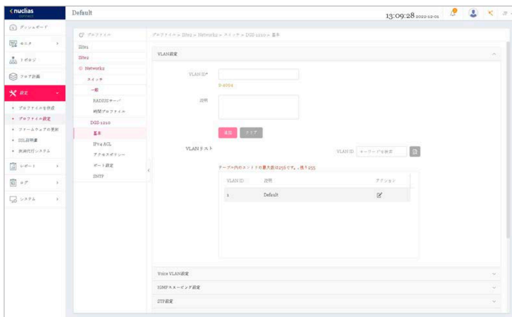
図 8-34 プロファイル設定 - スイッチ - 基本 (VLAN)
