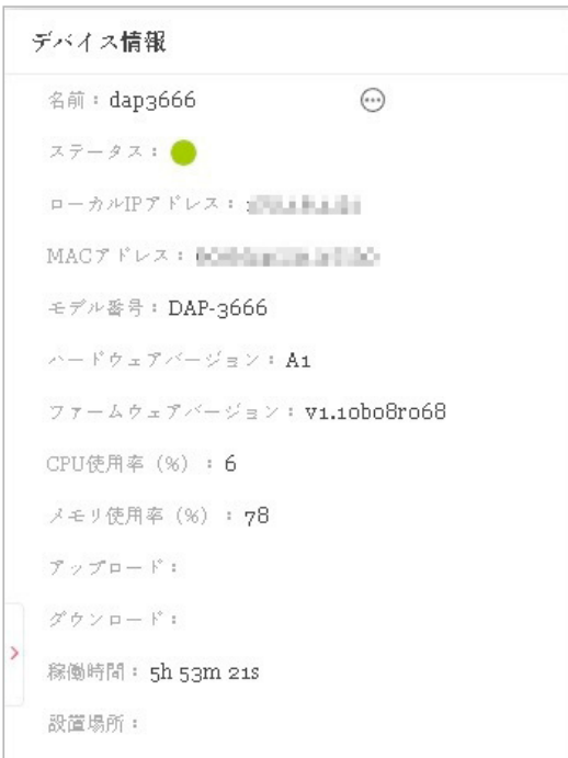
図 6-2 デバイス情報
