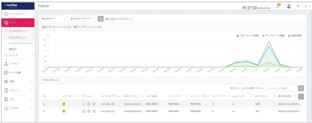
図 5-1 モニタ - アクセスポイント - アクセスポイント
