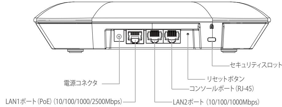
図 2-24 DBA-X5480P 背面パネル
