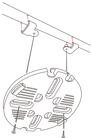
図 3-41 DBA-X2830P ブラケットとマウントプレートの取り付け
