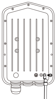
図 3-36 DBA-3621P アース線の接続
