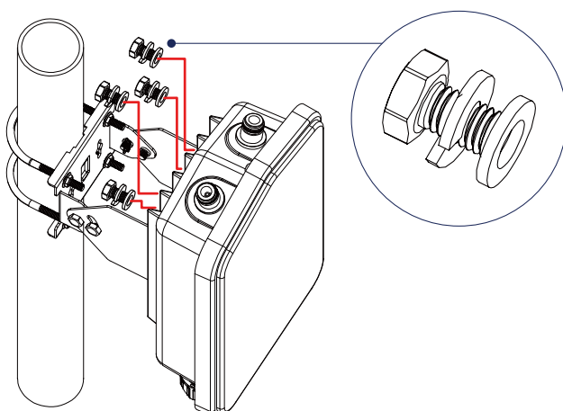
図 3-33 DBA-3621P 柱用マウントプレートへの取り付け
