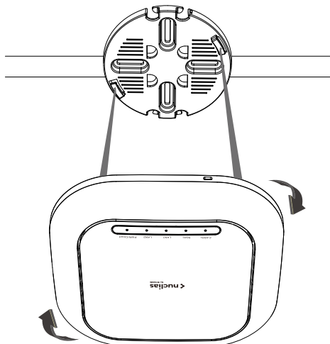
図 3-29 DBA-2820P マウントプレートへの取り付け
