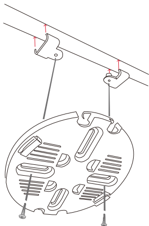
図 3-18 DBA-2620P ブラケットとマウントプレートの取り付け
