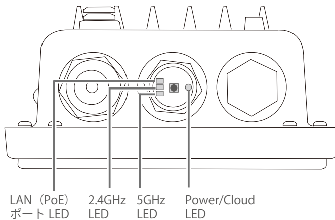
図 2-17 DBA-3621P LED 表示
