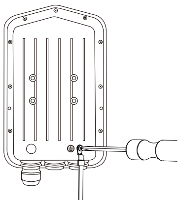
図 3-37 DBA-3621P アース線の固定
