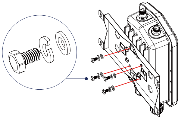
図 3-34 DBA-3621P マウントプレートの取り付け
