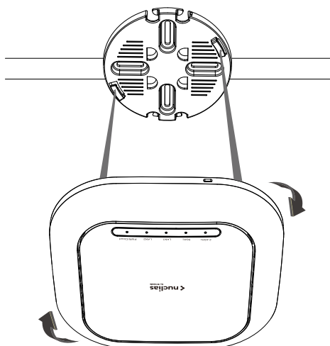
図 3-24 DBA-2720P マウントプレートへの取り付け
