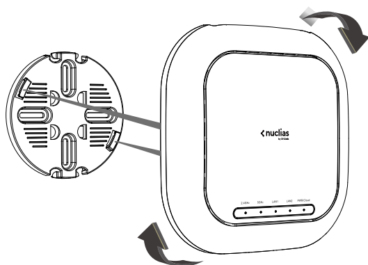
図 3-40 DBA-X2830P マウントプレートへの取り付け
