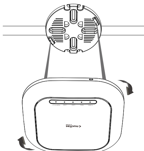
図 3-14 DBA-2520P マウントプレートへの取り付け
