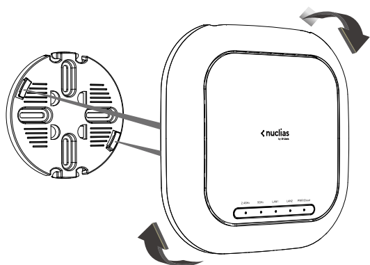
図 3-12 DBA-2520P マウントプレートへの取り付け
