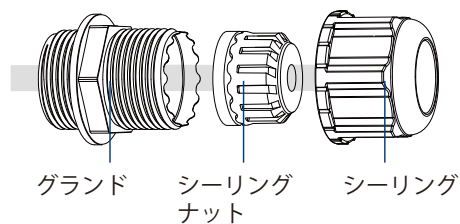
図 3-31 DBA-3621P 防水コネクタ
