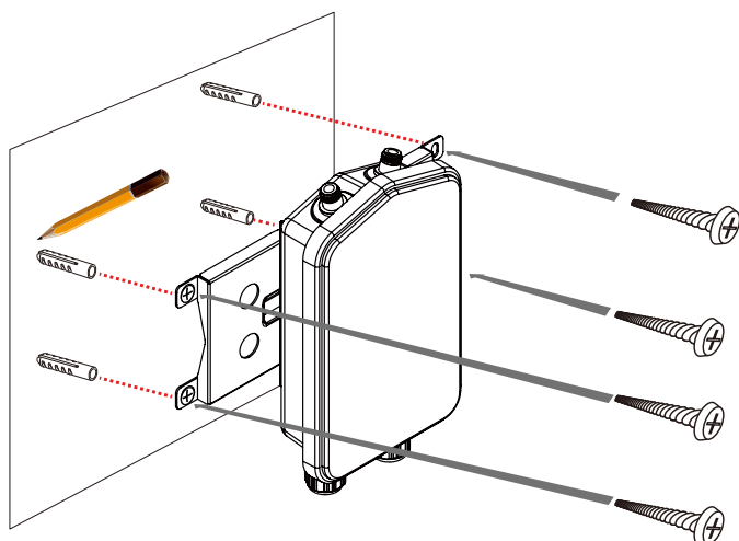
図 3-35 DBA-3621P 壁への取り付け
