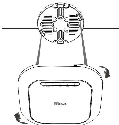
図 3-42 DBA-X2830P マウントプレートへの取り付け
