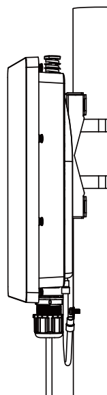
図 3-38 DBA-3621P アース線の取り付け
