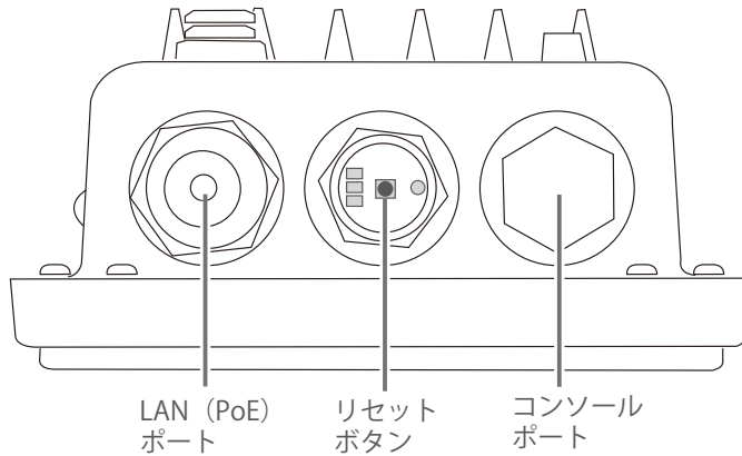
図 2-16 DBA-3621P 底面
