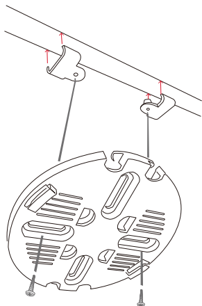
図 3-23 DBA-2720P ブラケットとマウントプレートの取り付け
