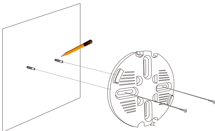
図 3-11 DBA-2520P 天井または壁面への設置
