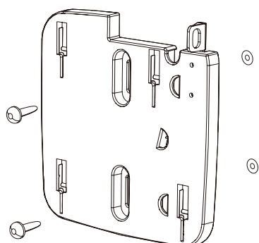
図 3-8 DBA-1210P マウントプレートネジ止め
