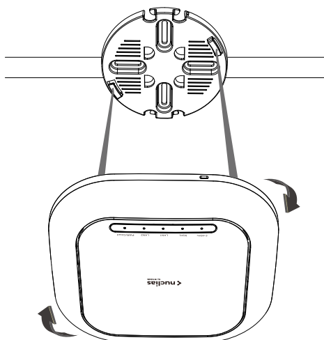
図 3-19 DBA-2620P マウントプレートへの取り付け
