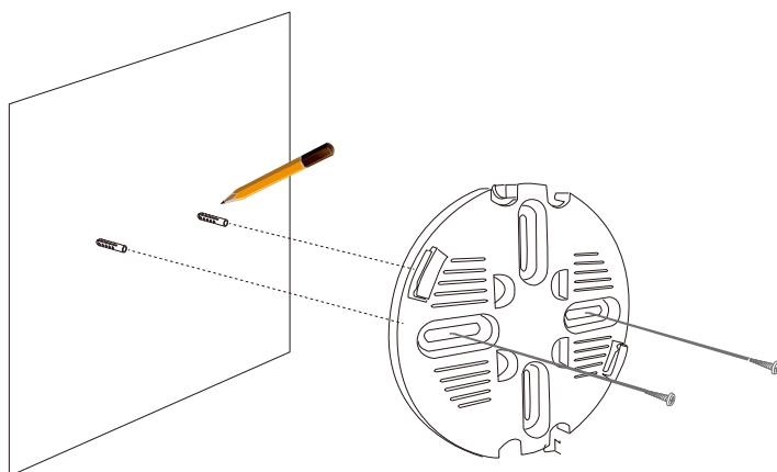
図 3-16 DBA-2620P 天井または壁面への設置
