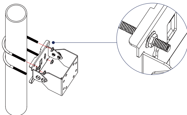
図 3-32 DBA-3621P 柱への設置
