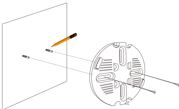
図 3-39 DBA-X2830P 天井または壁面への設置
