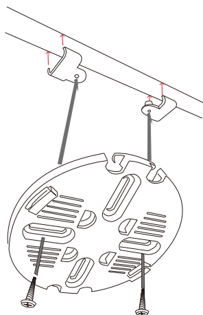
図 3-46 DBA-X1230P ブラケットとマウントプレートの取り付け
