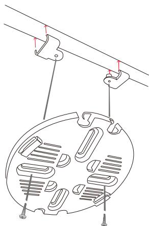
図 3-13 DBA-2520P ブラケットとマウントプレートの取り付け
