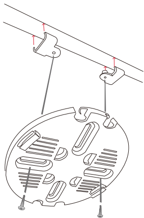
図 3-28 DBA-2820P ブラケットとマウントプレートの取り付け
