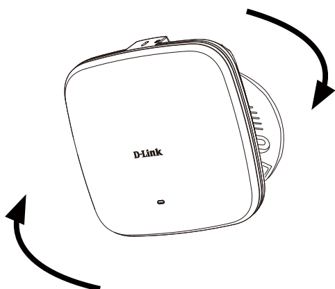
図 3-47 DBA-X1230P マウントプレートへの取り付け
