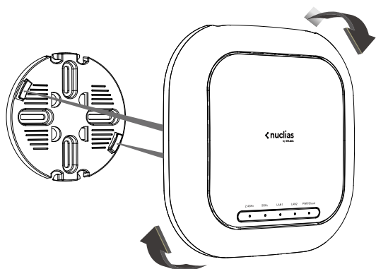
図 3-22 DBA-2720P マウントプレートへの取り付け
