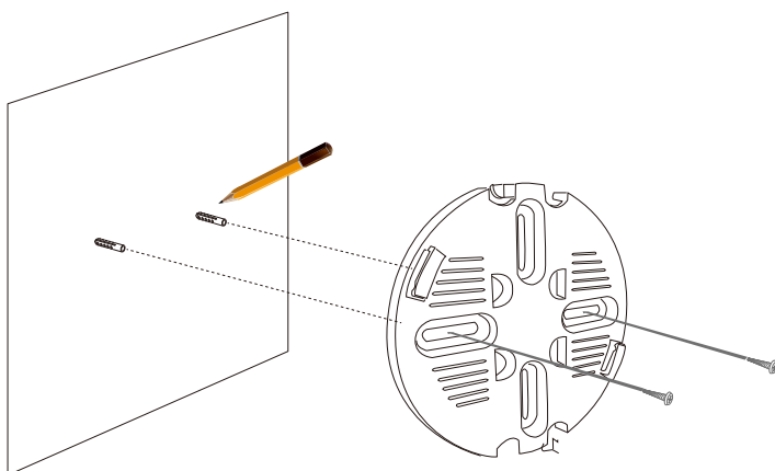
図 3-44 DBA-X1230P マウントプレートの取り付け
