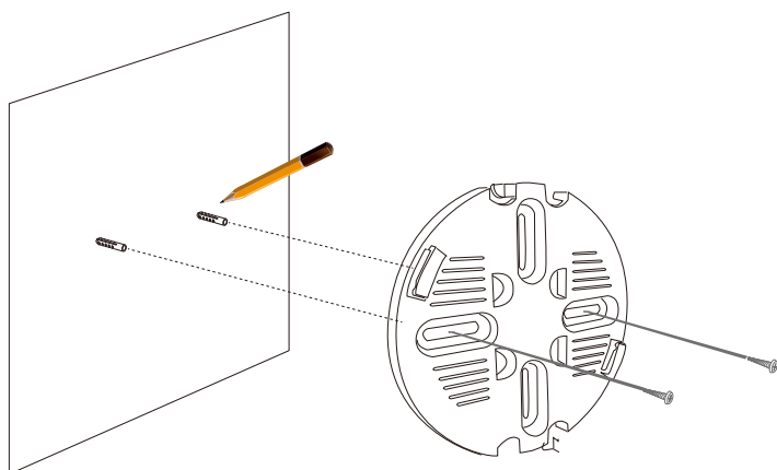
図 3-21 DBA-2720P 天井または壁面への設置
