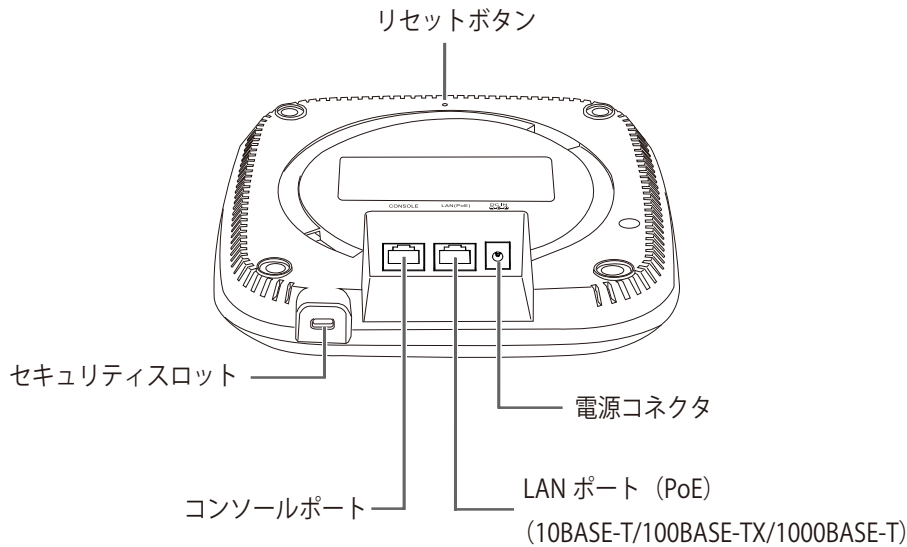
図 2-22 DBA-X1230P 背面パネル
