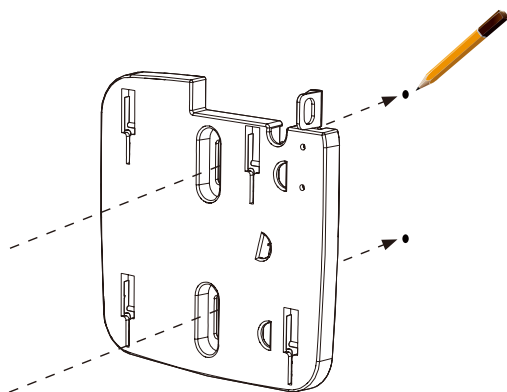
図 3-6 DBA-1210P 位置確認（壁面設置）
