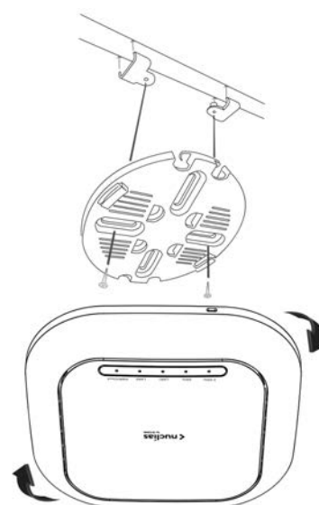
図 3-13 DBA-2520P 天井クロスバーへの設置
