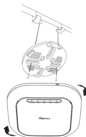
図 3-21 DBA-2720P 天井クロスバーへの設置
