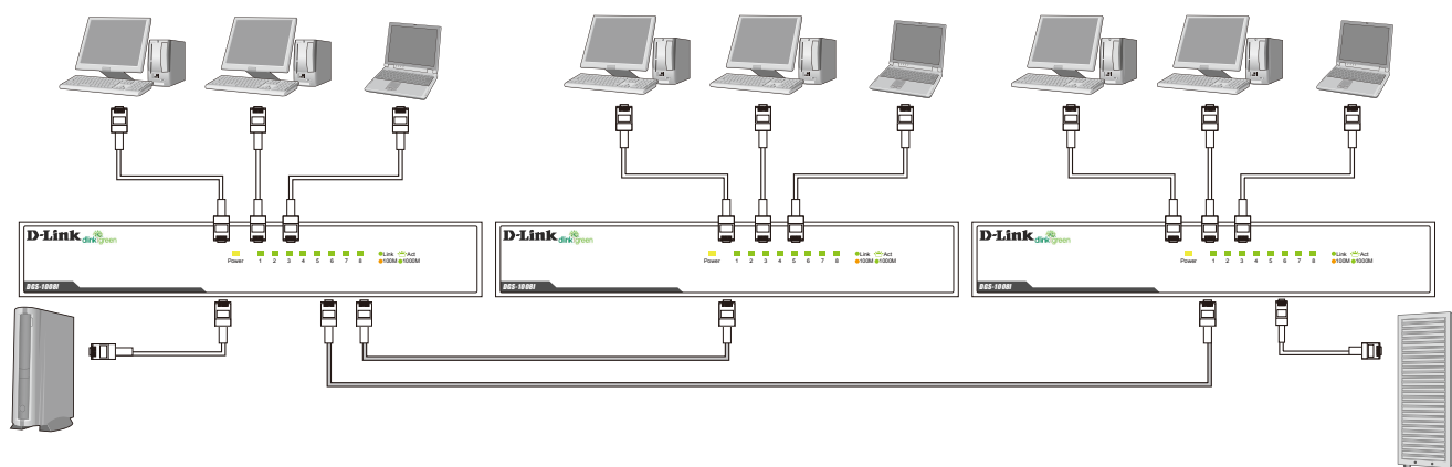
図 3-2 カスケード接続
