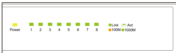
図 1-4 DGS-1008I/RM の LED 配置図
