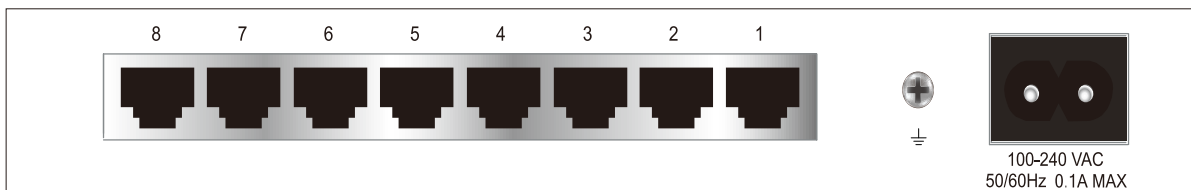
図 1-3 DGS・DES-1008I/RM の背面パネル図
