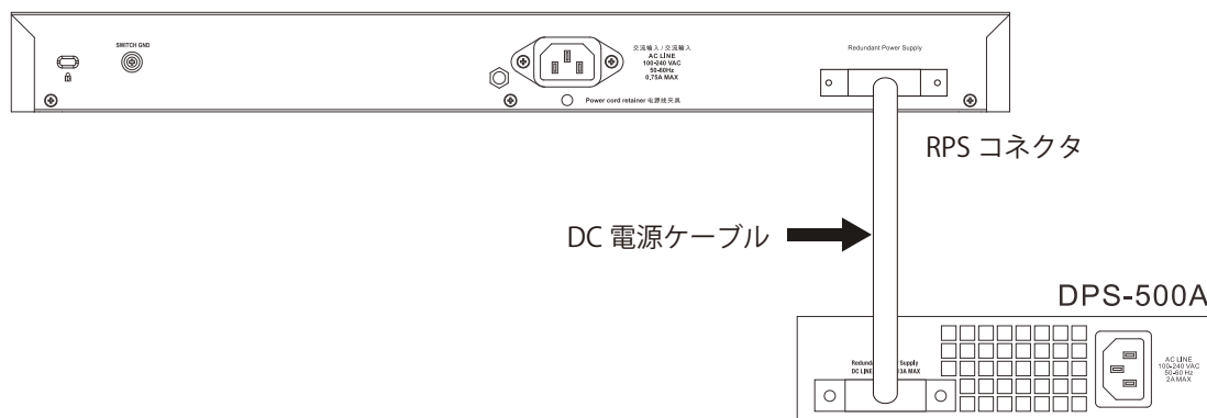
図 2-10 DGS-3630-28TC/SC と DPS-500A RPS の接続
