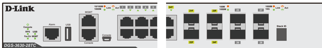
図 1-7 DGS-3630-28TC の前面パネル LED 配置図
