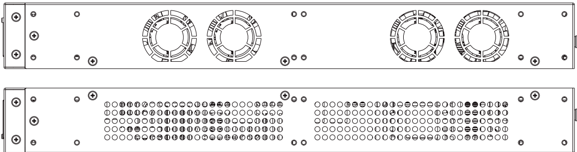
図 1-18 側面パネル図 (DGS-3630-28PC / DGS-3630-52PC)
