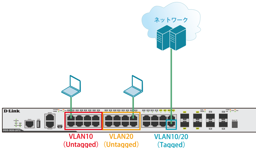
図 1-2 VLAN (DGS-3630-28TC)
