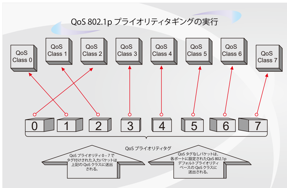
図 10-1 スイッチ上での QoS マッピングの例
