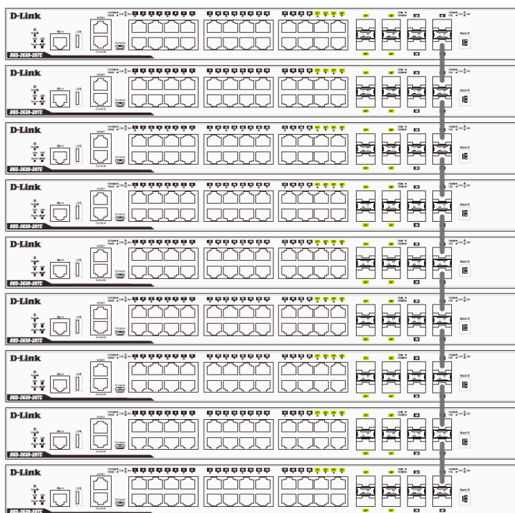
図 7-84 Duplex Chain でスタックされているスイッチ画面 (SFP +)
