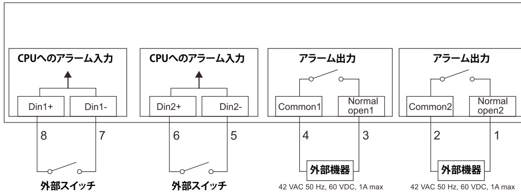
図 1-6 アラームコネクタ
