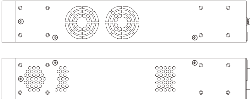
図 1-16 側面パネル図 (DGS-3630-28TC / DGS-3630-28SC)
