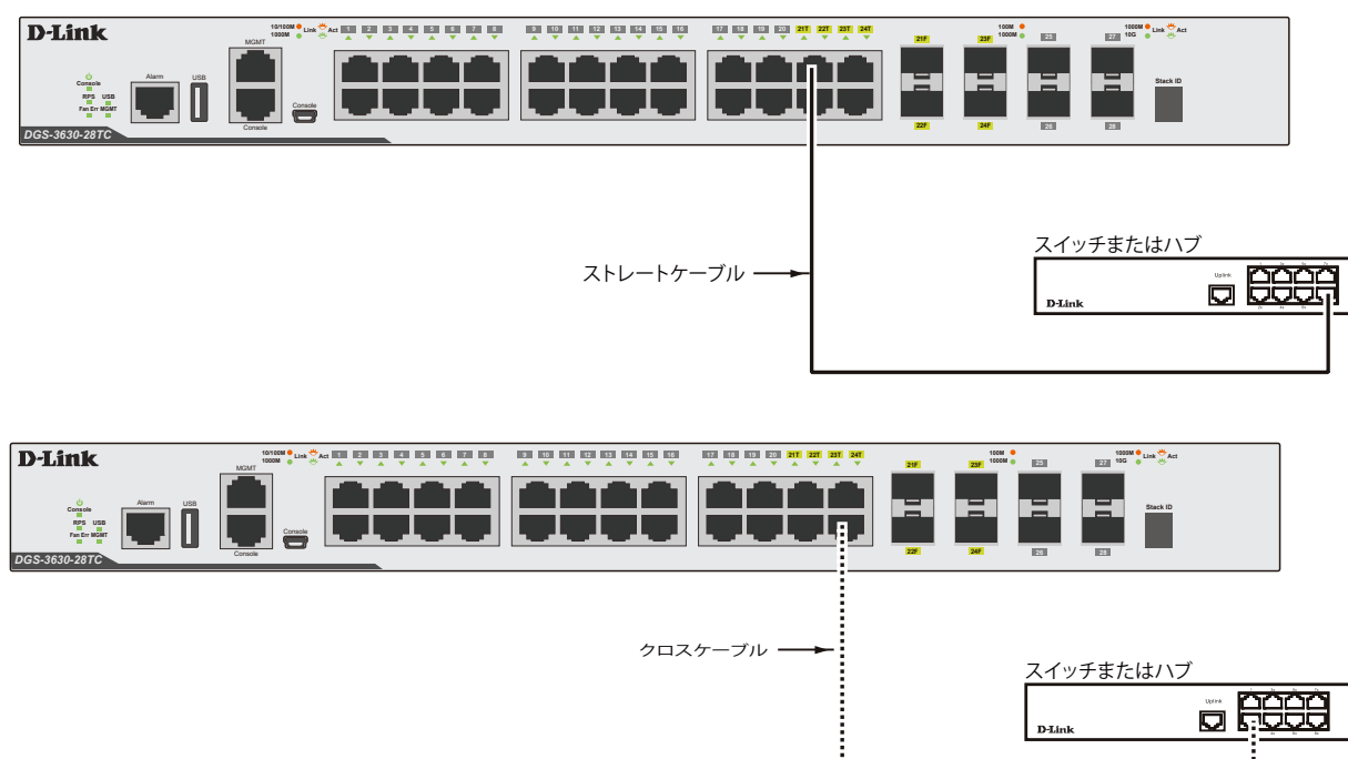
図 3-2 ストレート、クロスケーブルでハブまたはスイッチと接続する図
