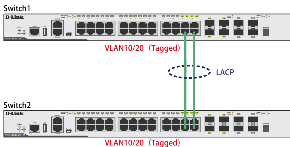
図 1-3 Link Aggregation (DGS-3630-28TC)
