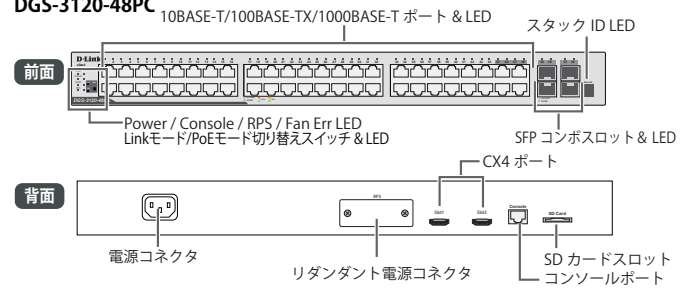
DGS-3120-48PC
