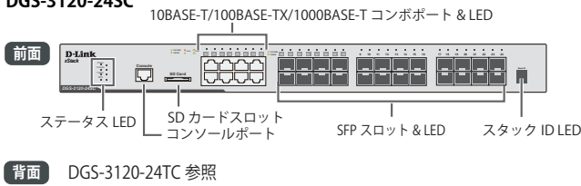
DGS-3120-24SC
