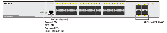
DGS-3000-28XMP
