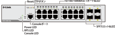
DGS-3000-28L
