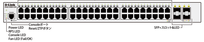
DGS-3000-52X
