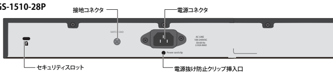
DGS-1510-28P
