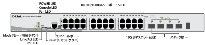
DGS-1510-28XMP
