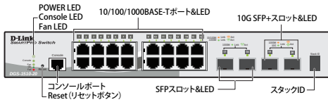
DGS-1510-28P
