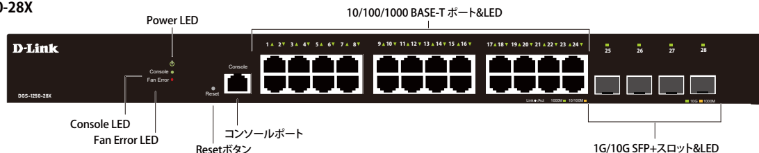
DGS-1250-28XP
