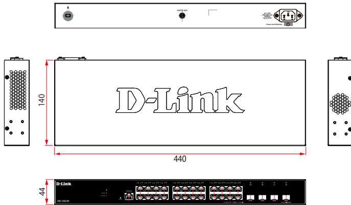
DGS-1250-28X
