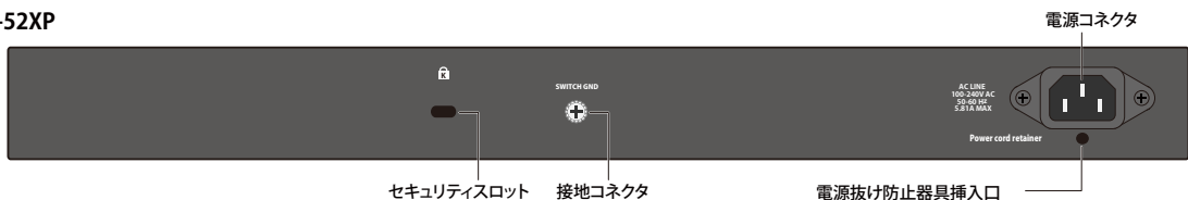
DGS-1250-52XP
