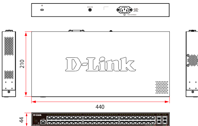
DGS-1250-52X
