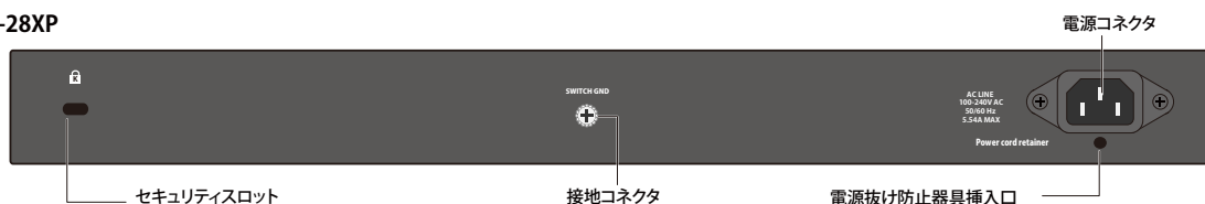
DGS-1250-28XP
