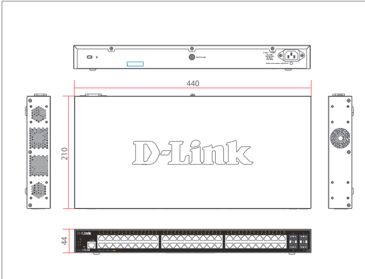
DGS-1250-52X
