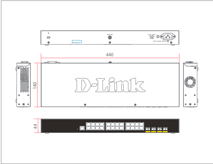
DGS-1250-28X
