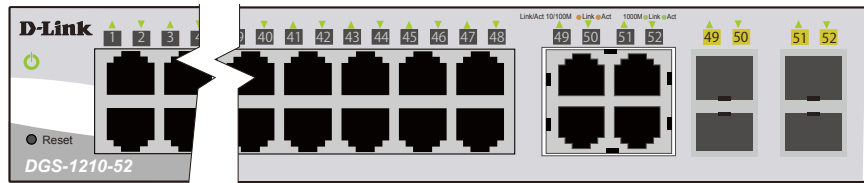
図 1-10 DGS-1210-52 の前面パネル LED 配置図
