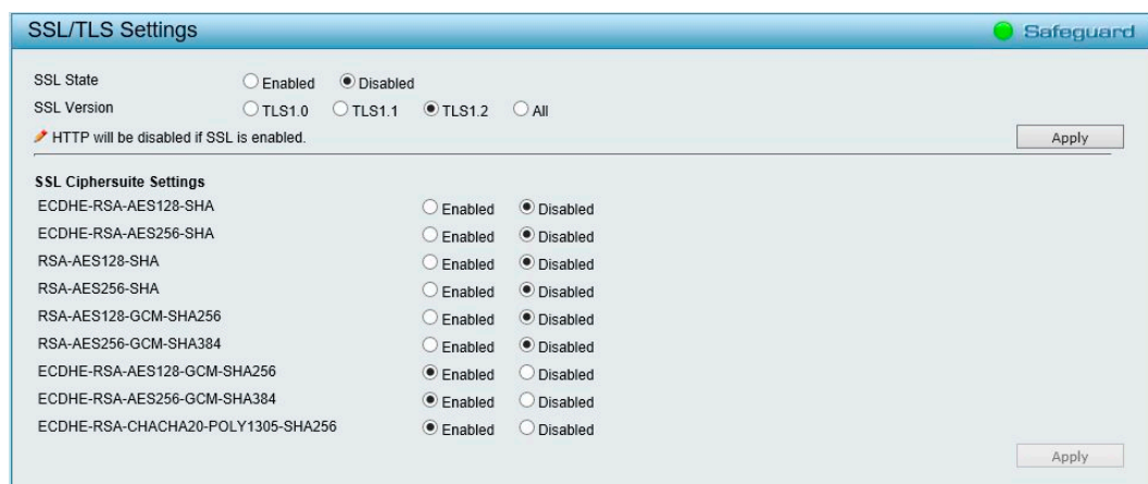
図 5-117 SSL/TLS Settings 画面
