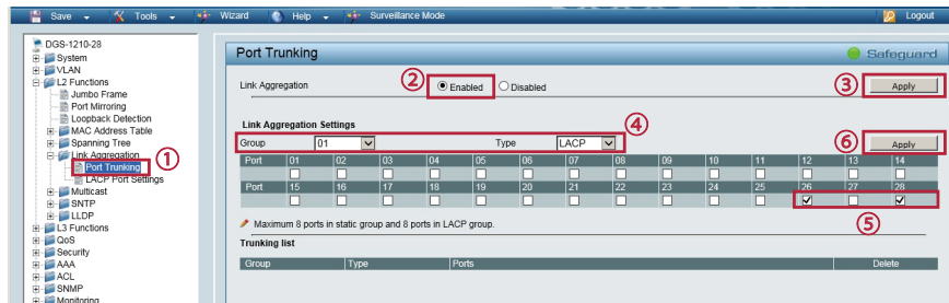
図 1-14 LACP 設定 (DGS-1210-28)
