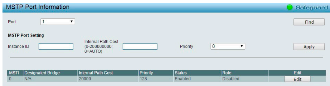
図 5-71 MSTP Port Information 画面
