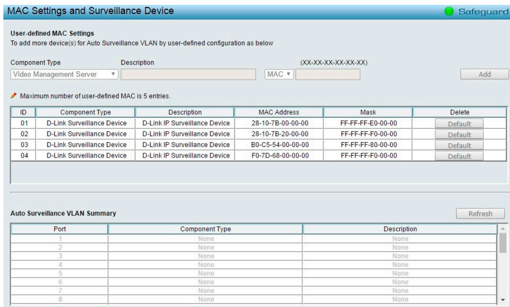
図 5-58 MAC Settings and Surveillance Device 画面
