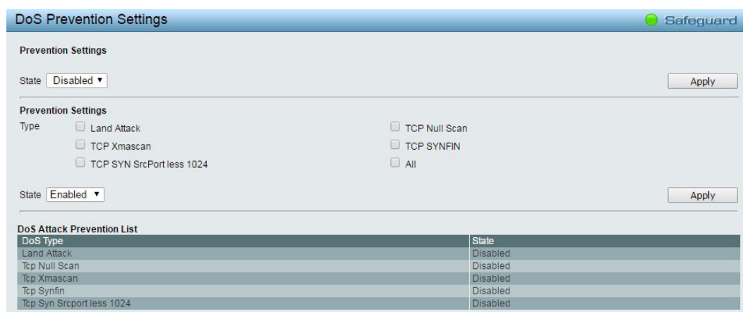
図 5-118 DoS Prevention Settings 画面
