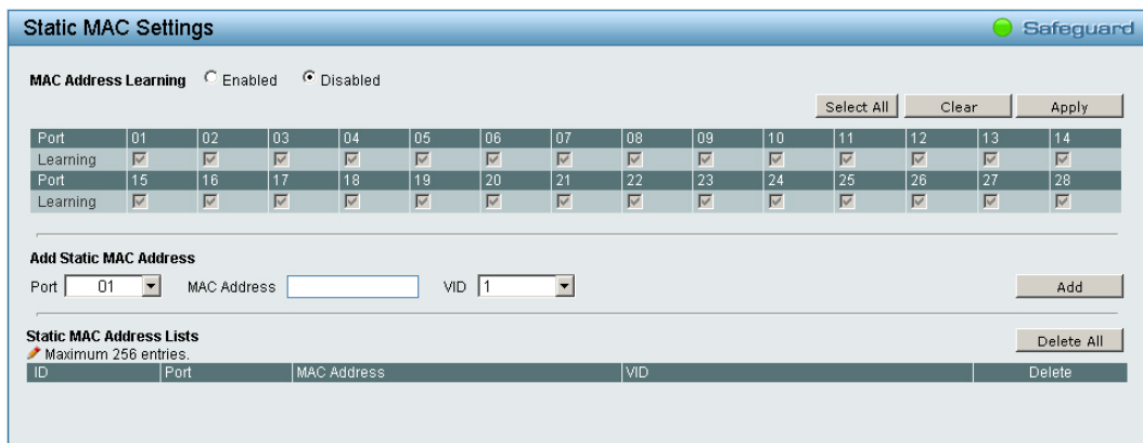
図 5-64 Static MAC Settings 画面
