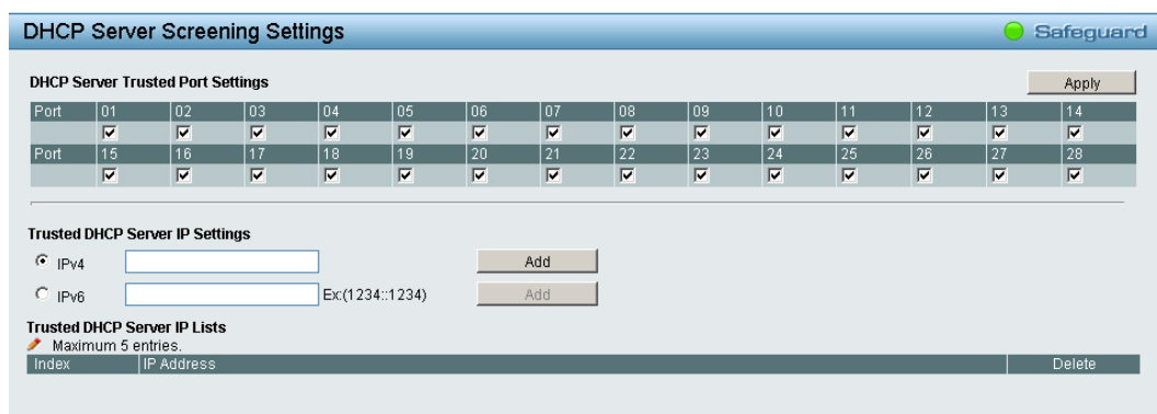
図 5-116 DHCP Server Screening Settings 画面
