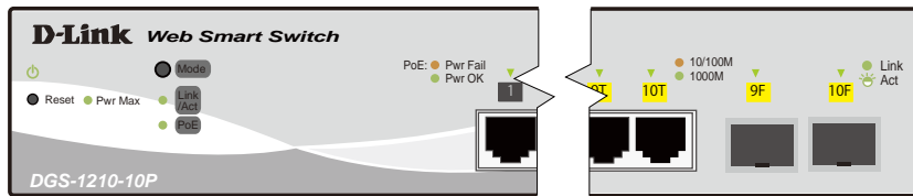
図 1-9 DGS-1210-10P の前面パネルの LED 配置図
