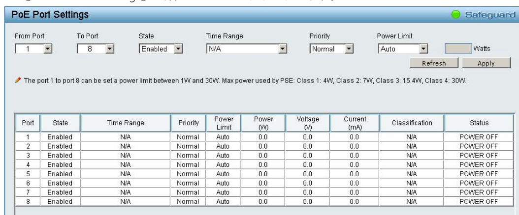
図 5-107 PoE Port Settings 画面
