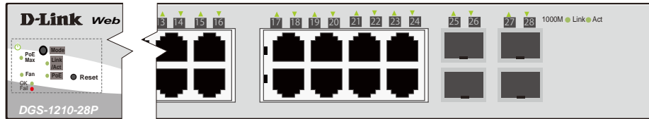
図 1-10 DGS-1210-28P の前面パネルの LED 配置図
