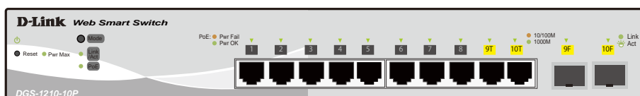
図 1-4 DGS-1210-10P の前面パネル図
