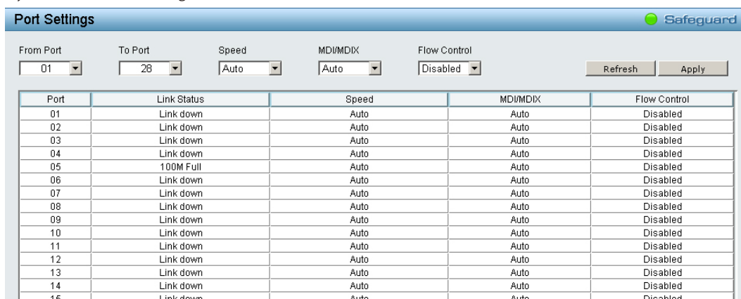
図 5-29 Port Settings 画面
