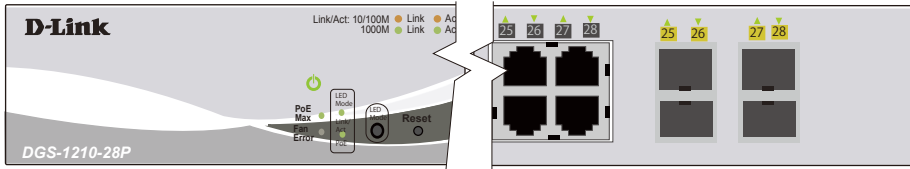
図 1-12 DGS-1210-28P の前面パネルの LED 配置図
