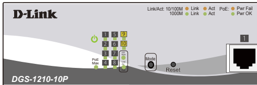
図 1-11 DGS-1210-10P の前面パネルの LED 配置図
