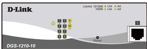
図 1-7 DGS-1210-10 の前面パネルの LED 配置図
