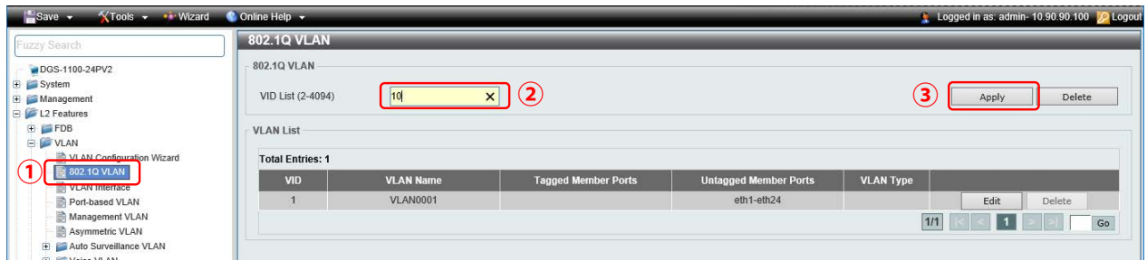
図 16-15 VLAN 作成
