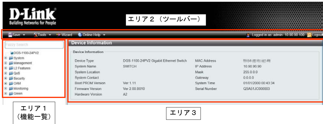
図 5-7 初期画面
