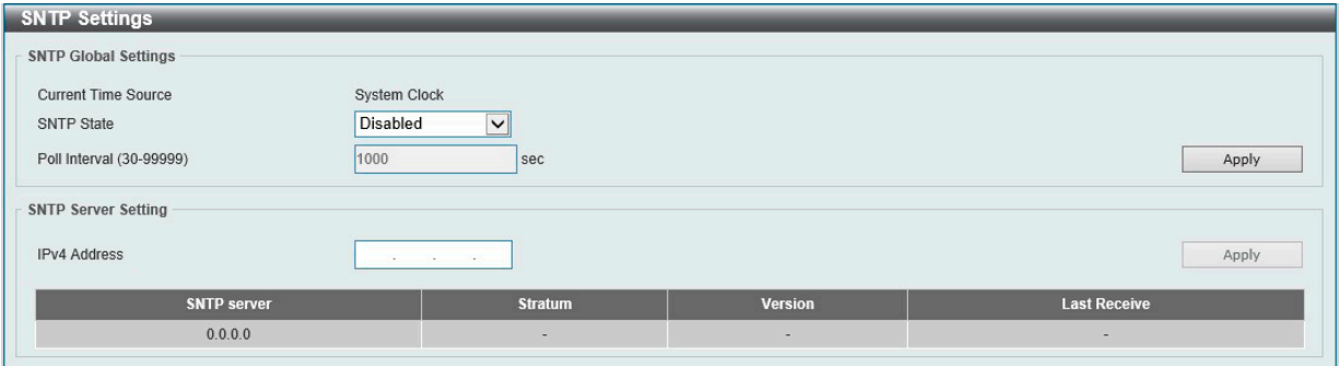
図 6-17 SNTP Settings 画面
