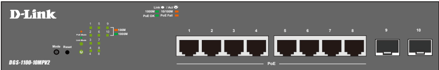
図 1-4 DGS-1100-10MPV2 の前面パネル図
