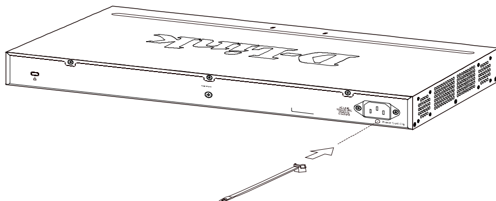
図 2-4 タイラップの挿し込み
