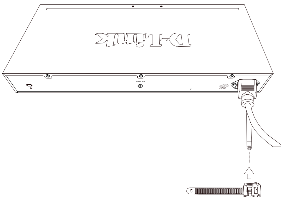
図 2-6 リテーナー（固定具）のスライド
