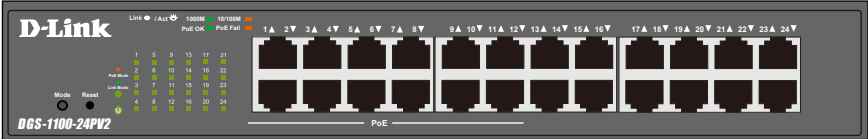
図 1-3 DGS-1100-24PV2 の前面パネル図
