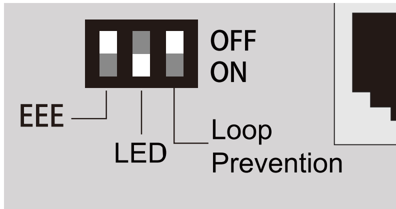
図 1-1 DIP スイッチ 図
