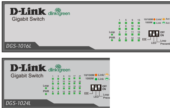
図 1-6 DGS-1016L、DGS-1024L の LED 配置図
