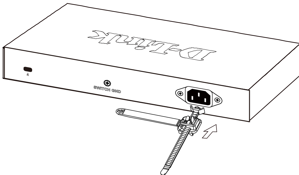
図 1-6 タイラップの挿し込み
