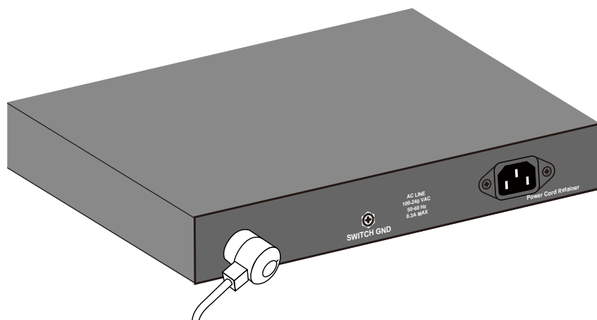
図 1-3 セキュリティロック設置
