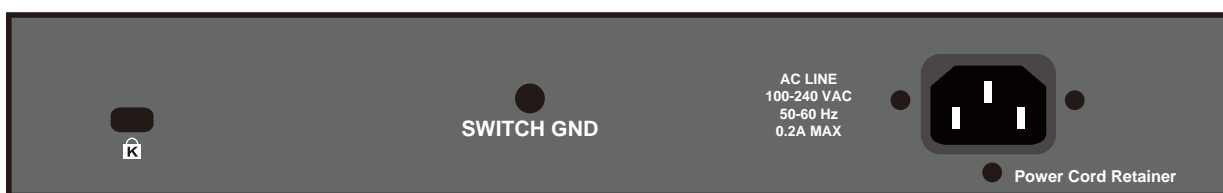
図 1-3 DGS-1016L の背面パネル図
