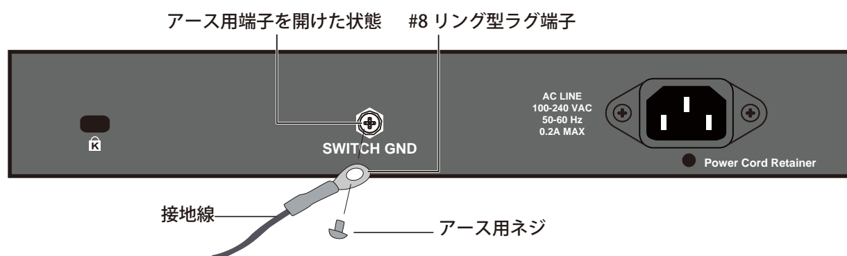
図 1-1 スwitchへのラグ端子の接地
