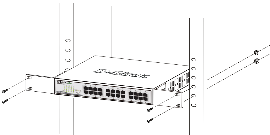
図 1-5 スイッチのラックへの設置
