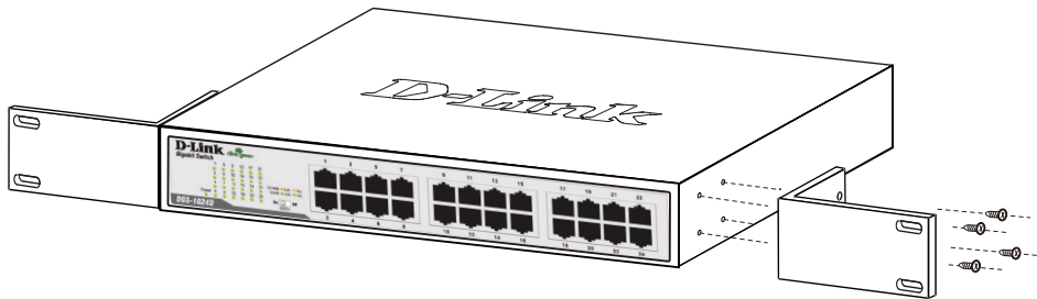
図 1-4 スイッチへのブラケットの取り付け
