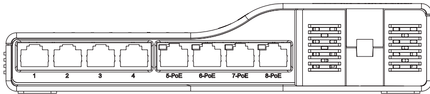
図 1-2 DGS-1008PTP の前面パネル図
