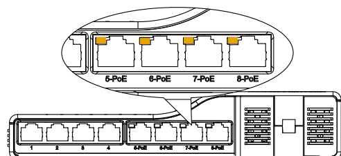
図 1-7 DGS-1008PTP の LED 配置図 (前面パネル)
