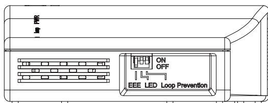
図 1-4 DGS-1008PTP の側面パネル図
