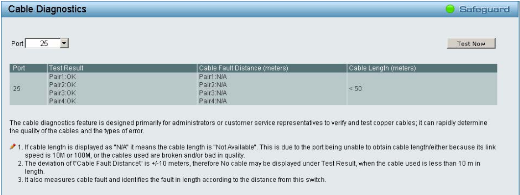
図 5-122 Cable Diagnostics 画面
