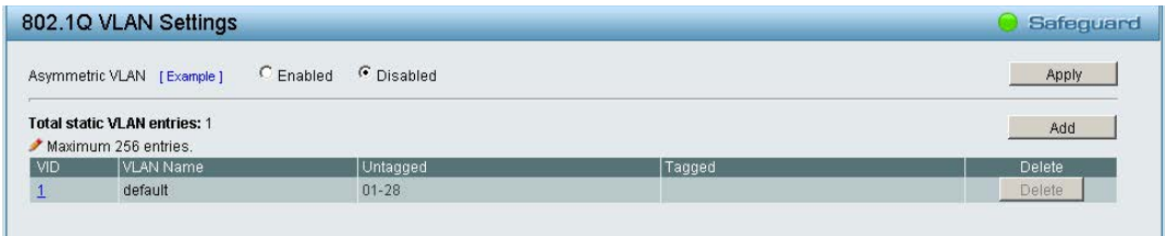
図 5-36 802.1Q VLAN Settings 画面
