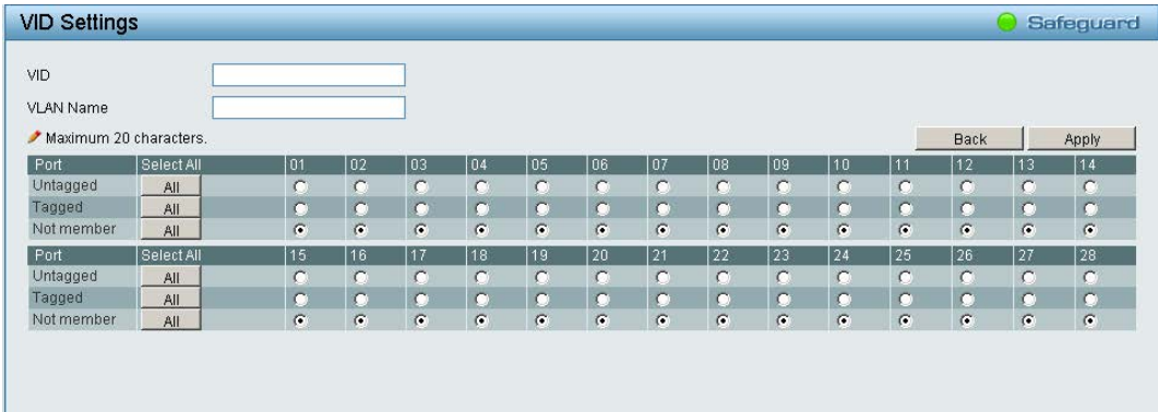
図 5-37 VID Settings 画面
