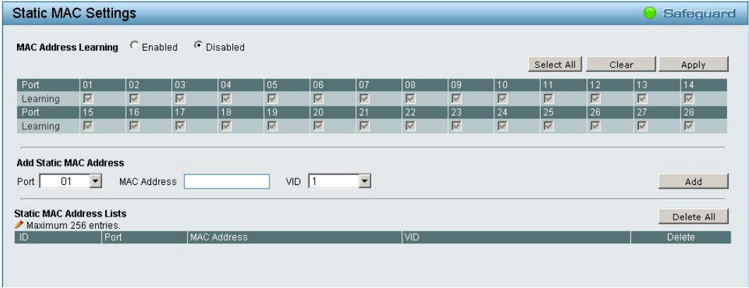
図 5-47 Static MAC Settings 画面
