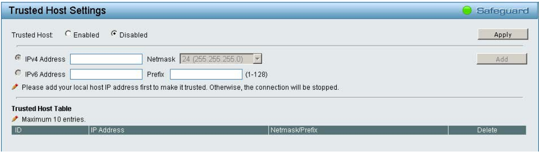
図 5-79 Trusted Host Settings 面
