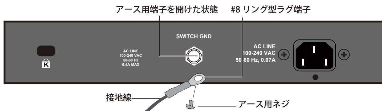
図 2-7 スwitchへのラグ端子の接地
