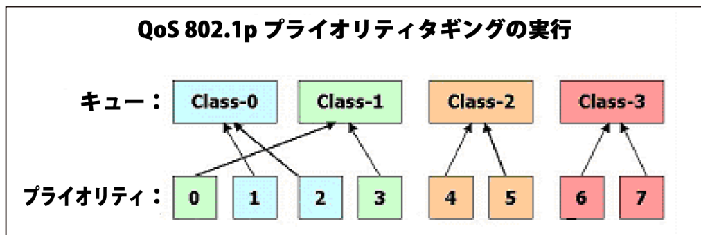
図 1-8 DES-1016D の QoS について
