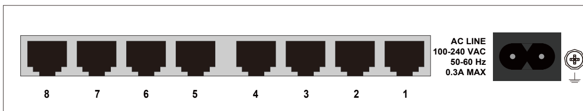
図 1-2 DES-1008I/ET の背面パネル図
