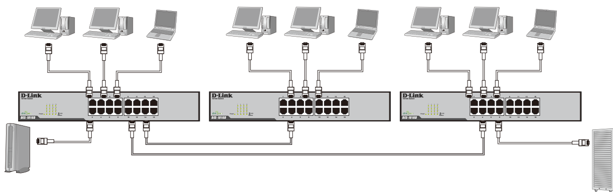
図 3-2 カスケード接続
