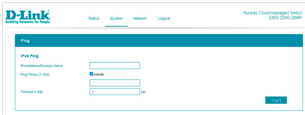
図 12-5 Ping 画面
