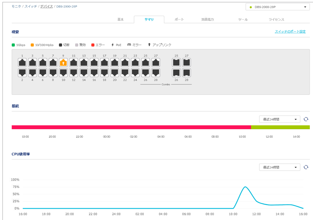
図 8-40 デバイス - サマリ
