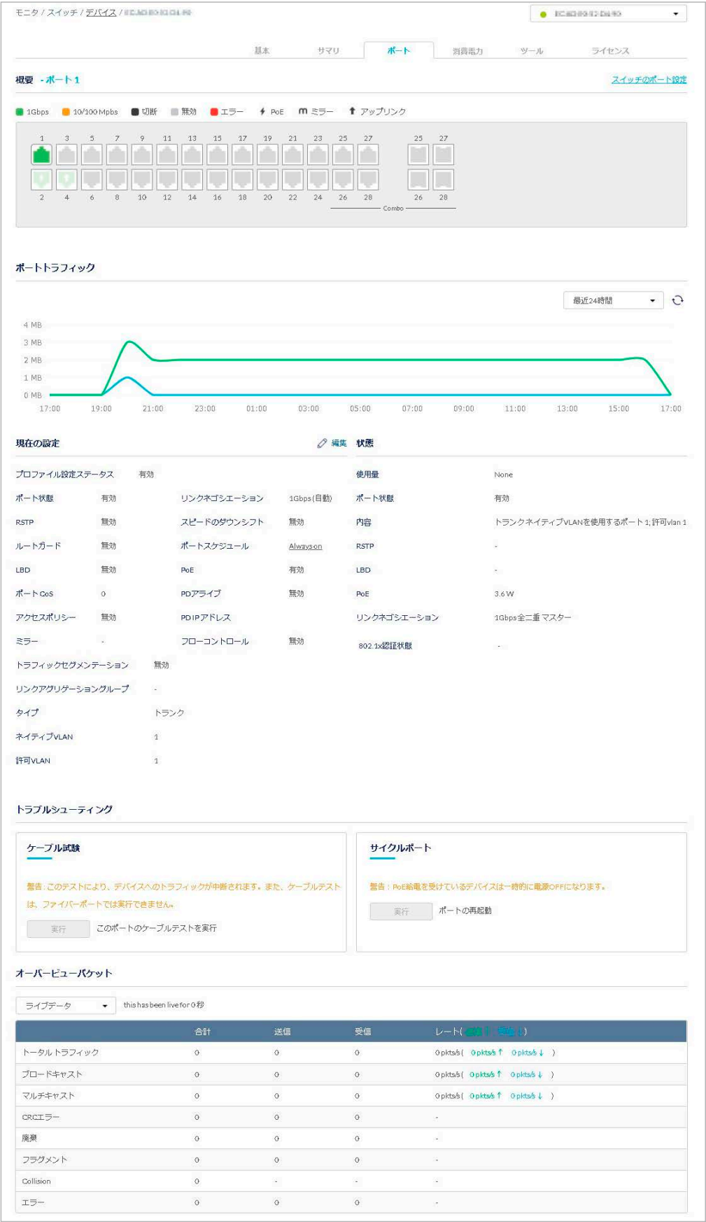
図 8-42 デバイス - ポート - ポート選択
