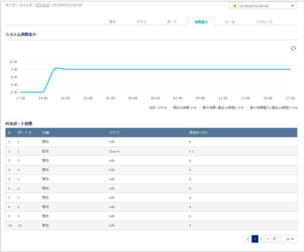
図 8-48 デバイス - 消費電力
