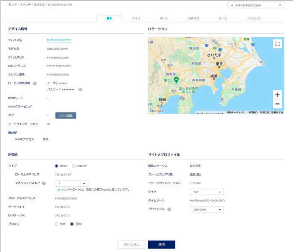
図 8-39 デバイス - 基本
