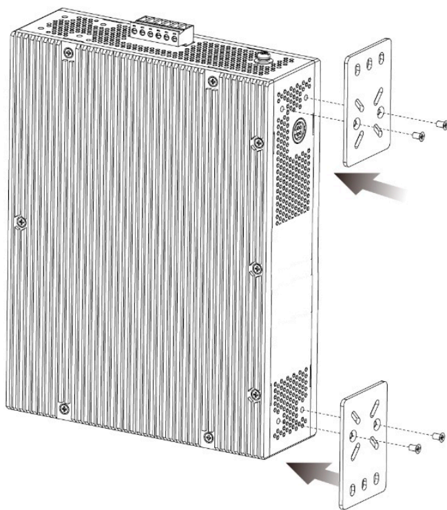
図 2-3 壁面取り付けプレートの取り付け
