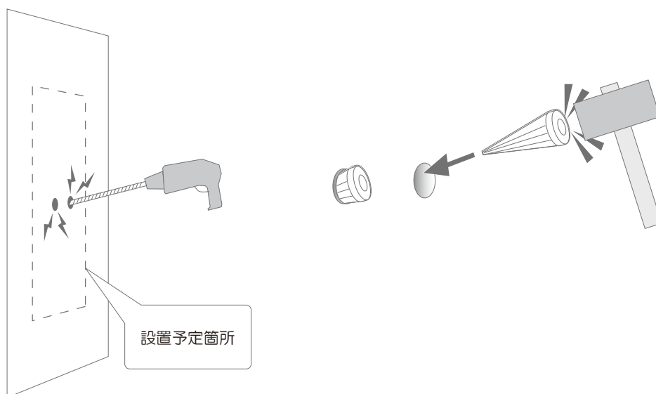
図 2-6 壁面への穴あけ、アンカー挿し込み
