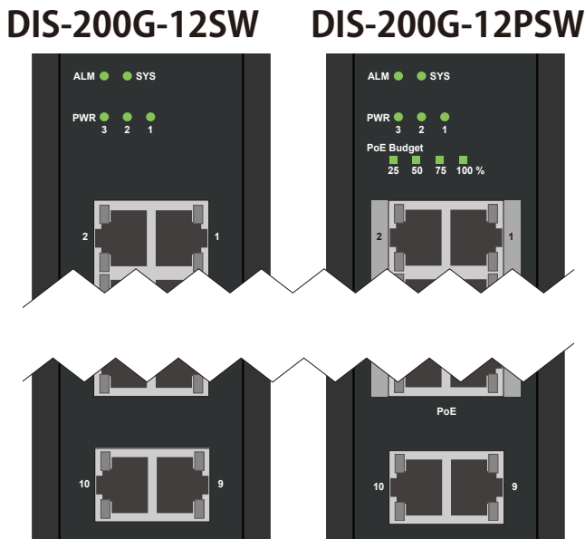
図 1-2 DIS-200G-12SW/12PSW 前面パネルの LED 配置図
