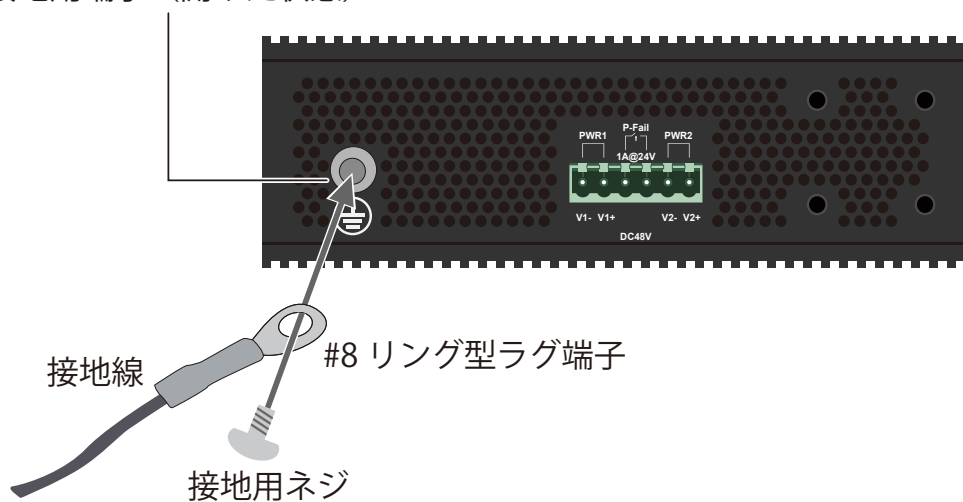
図 2-8 スwitchへのラグ端子の接地
