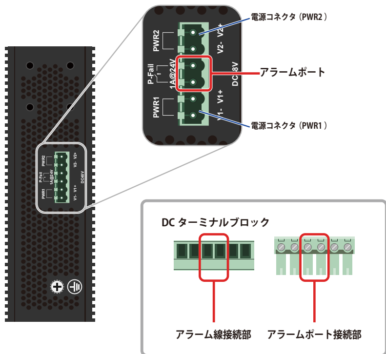
図 2-11 アラームポート
