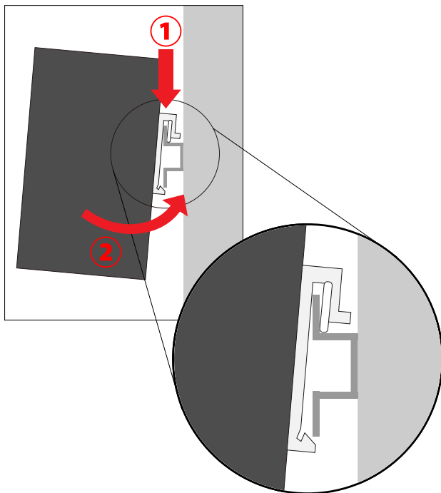
図 2-1 DIN レールへの設置
