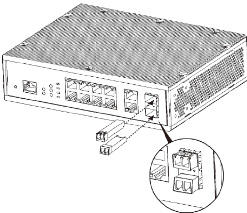
図 2-9 SFP モジュールの取り付け
