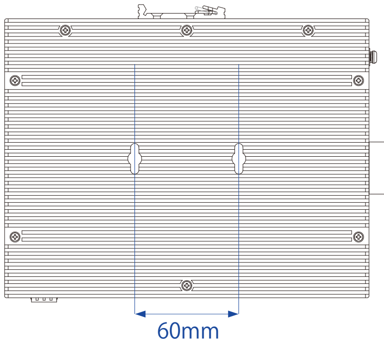
図 2-5 ネジ穴間隔
