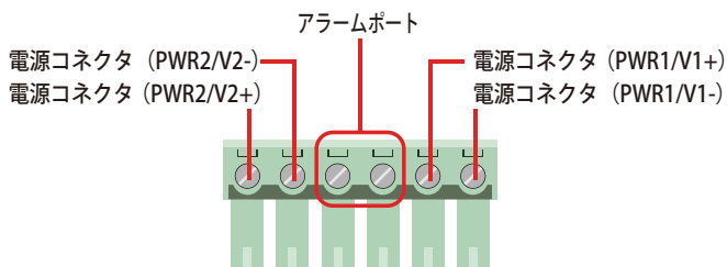
図 2-13 DC ターミナルブロックの接続端子部のネジと対応するコネクタ / ポート
