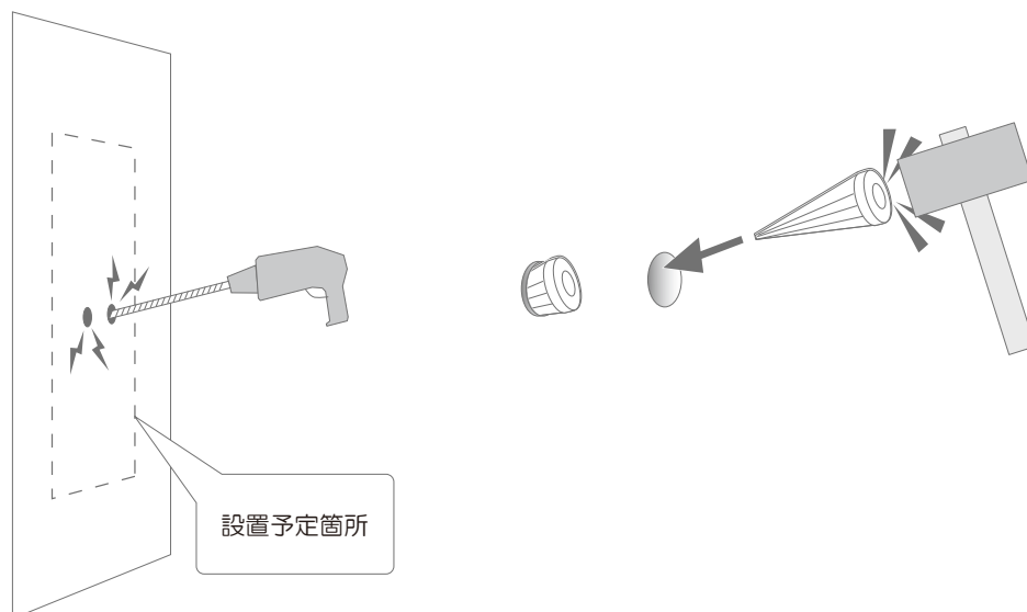
図 2-4 壁面への穴あけ、アンカー挿し込み
