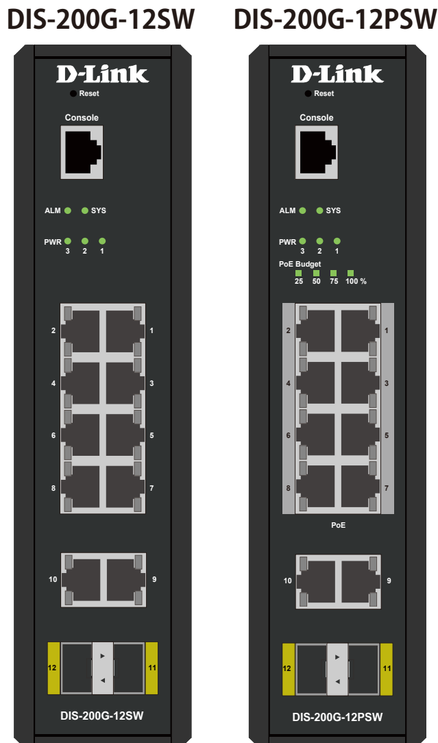
図 1-1 DIS-200G-12SW/12PSW 前面パネル図
