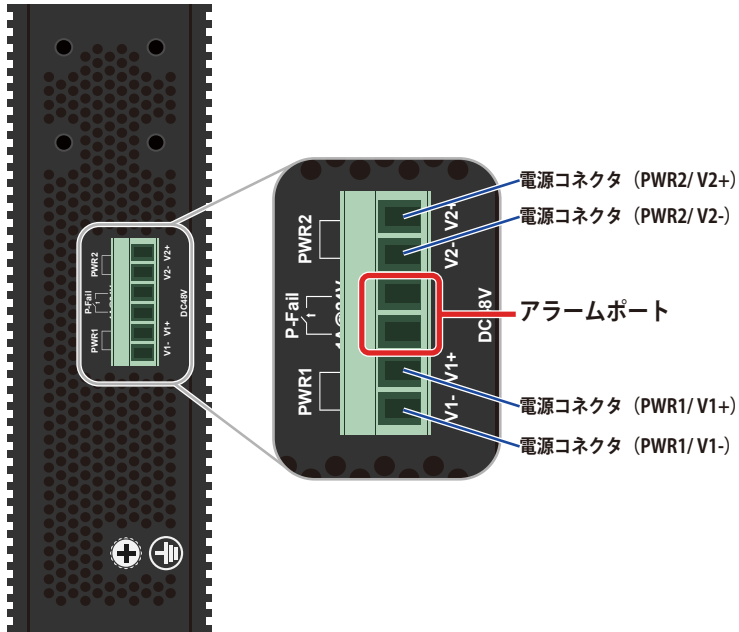
図 2-12 DC 電源コネクタ (DC ターミナルブロック接続時)
