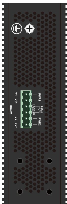
図 1-4 DIS-200G-12SW/12PSW の上面パネル図
