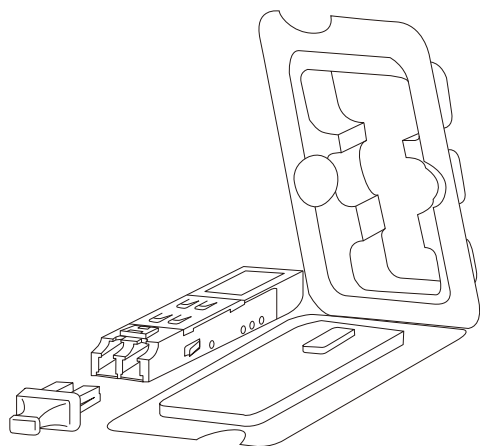
図 2-10 SFP モジュール図
