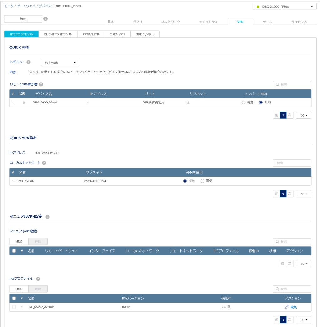
図 9-73 SITE TO SITE VPN
