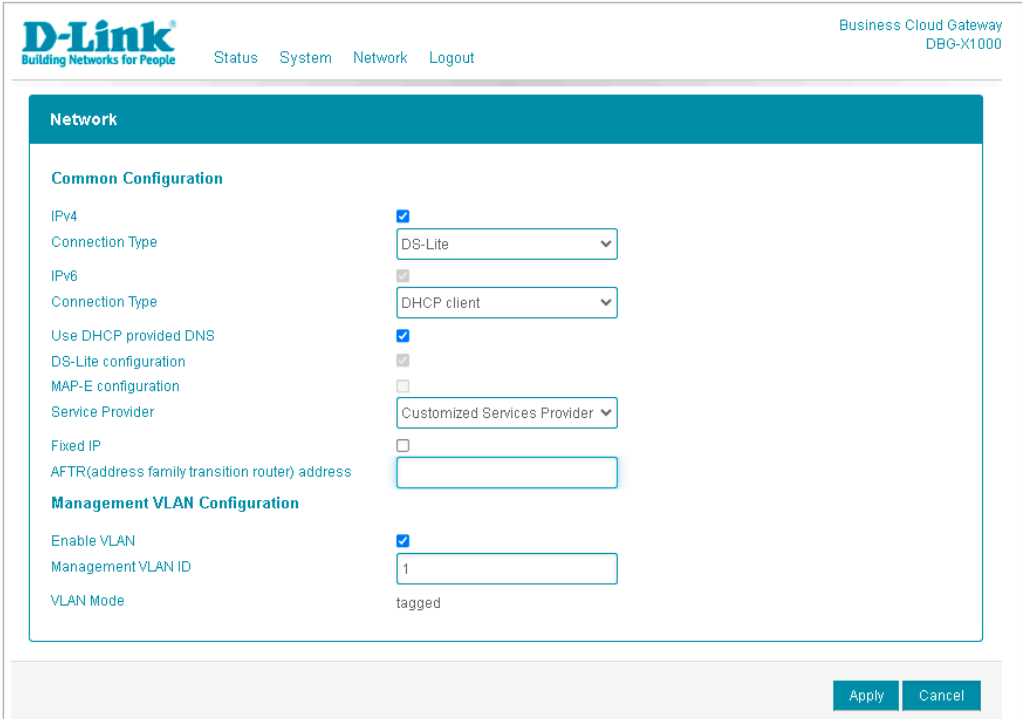
図 4-20 DBG-X1000 ネットワーク - 基本設定（DS-Lite 選択時）
