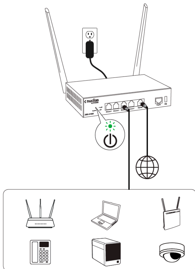
図 3-4 DBG-X1000 接続図
