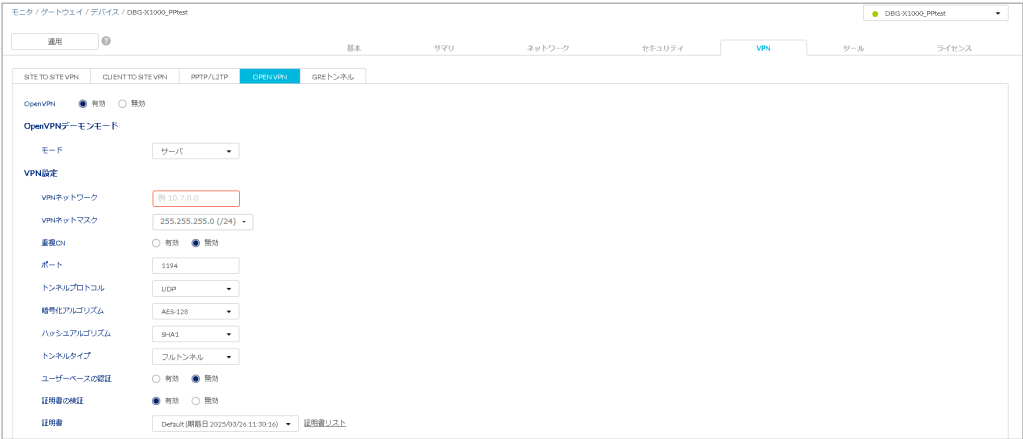
図 9-94 OPEN VPN（サーバモード）
