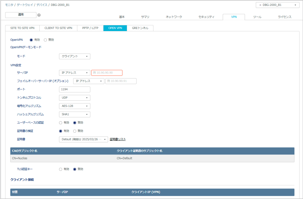
図 9-101 OPEN VPN（クライアントモード）
