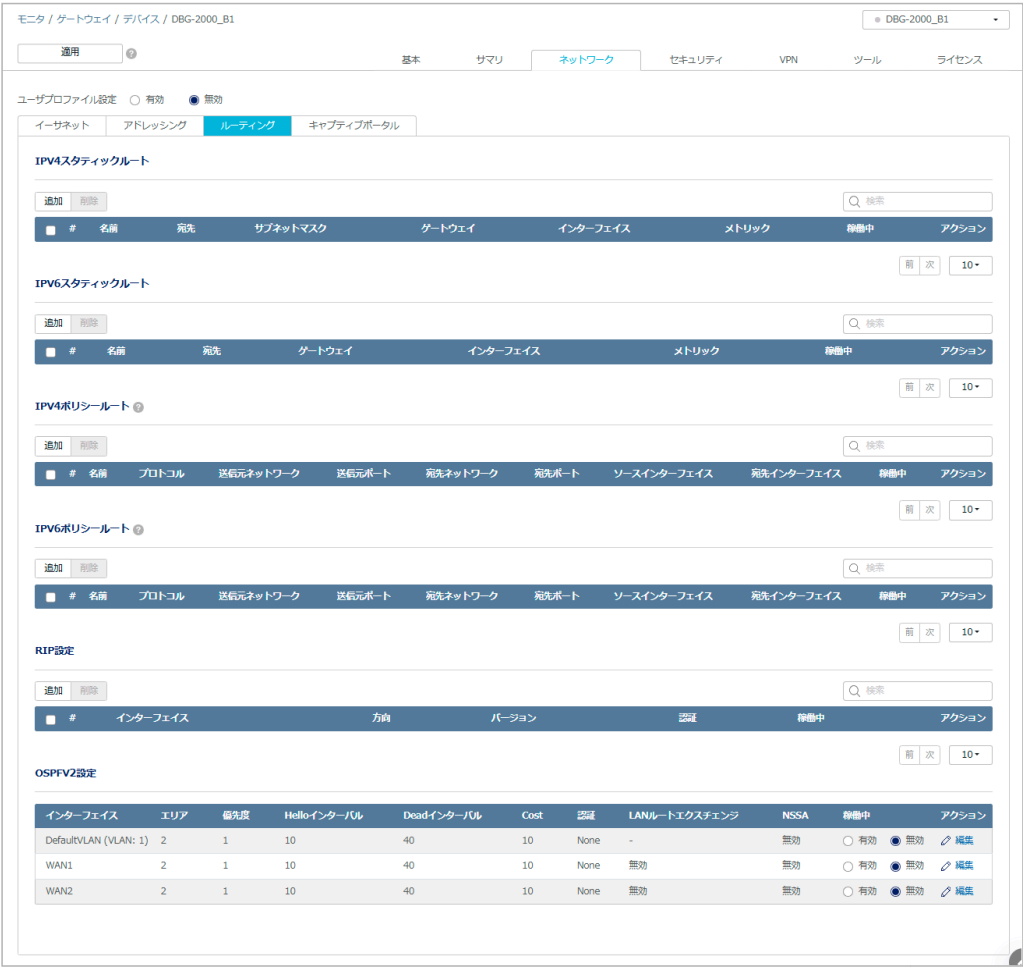
図 9-32 ルーティング
