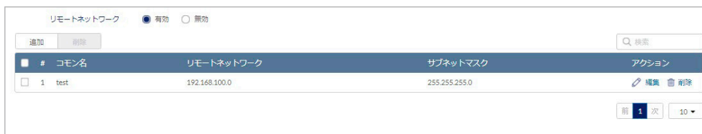
図 9-101 OPEN VPN (サーバモード) - リモートネットワーク
