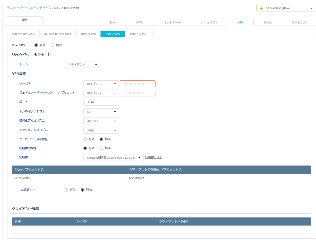
図 9-105 OPEN VPN (クライアントモード)
