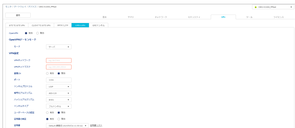
図 9-98 OPEN VPN (サーバモード)
