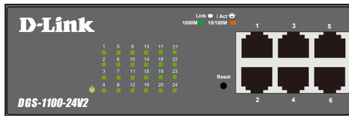
図 1-9 DGS-1100-24V2 の前面パネルの LED 配置図
