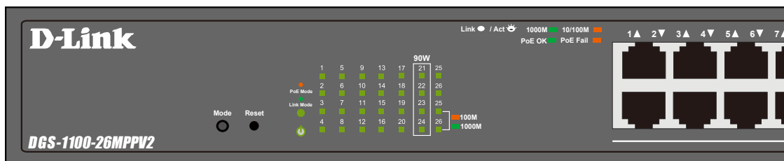
図 1-14 DGS-1100-26MPPV2 の前面パネルの LED 配置図
