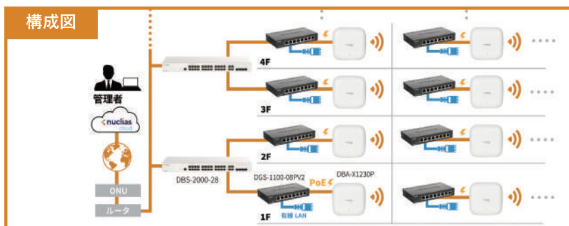
▲客室 Wi-Fi 設備の構成図。L2 スイッチの DBS-2000-28 が1台で2階分を担うフロアスイッチとして設置され、各部屋に DGS-1100-08PV2 が1台、無線 AP の DBA-X1230P が1台（広い部屋だと1台以上）取り付けられている
