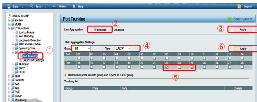
図 1-14 LACP 設定 (DES-1210-28)
