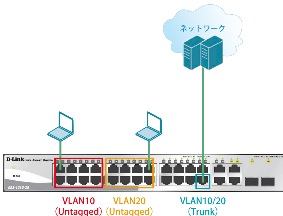
図 1-5 VLAN (DES-1210-28)
