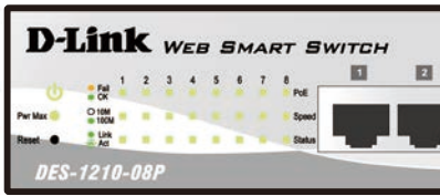
図 1-5 DES-1210-08P の前面パネルの LED 配置図
