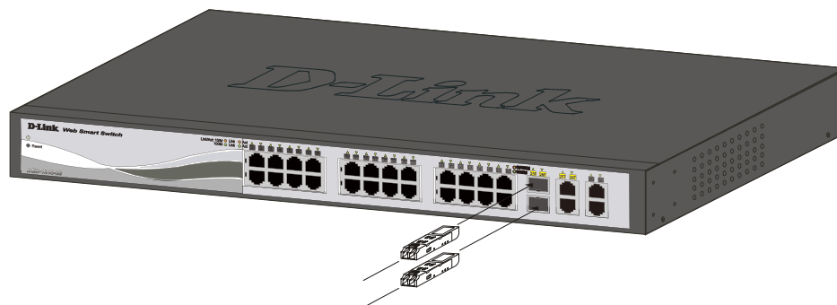
図 1-13 スイッチに光トランシーバを取り付ける
