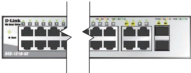
図 1-8 DES-1210-52 の前面パネルの LED 配置図
