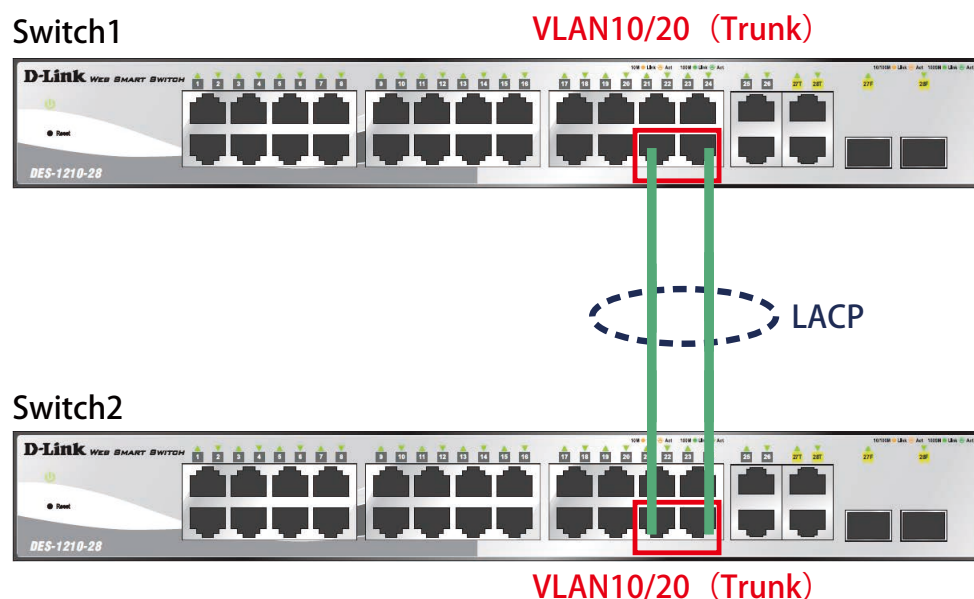
図 1-11 Link Aggregation（DES-1210-28）
