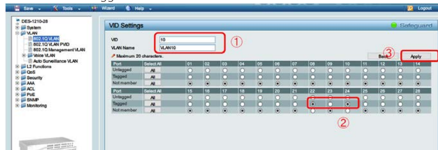
図 1-13 ポートアサイン（DES-1210-28）
