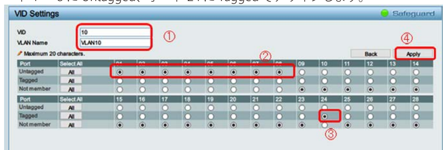
図 1-9 ポートアサイン (DES-1210-28)
