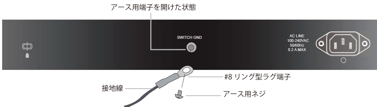
図 2-9 スイッチへのラグ端子の接続
